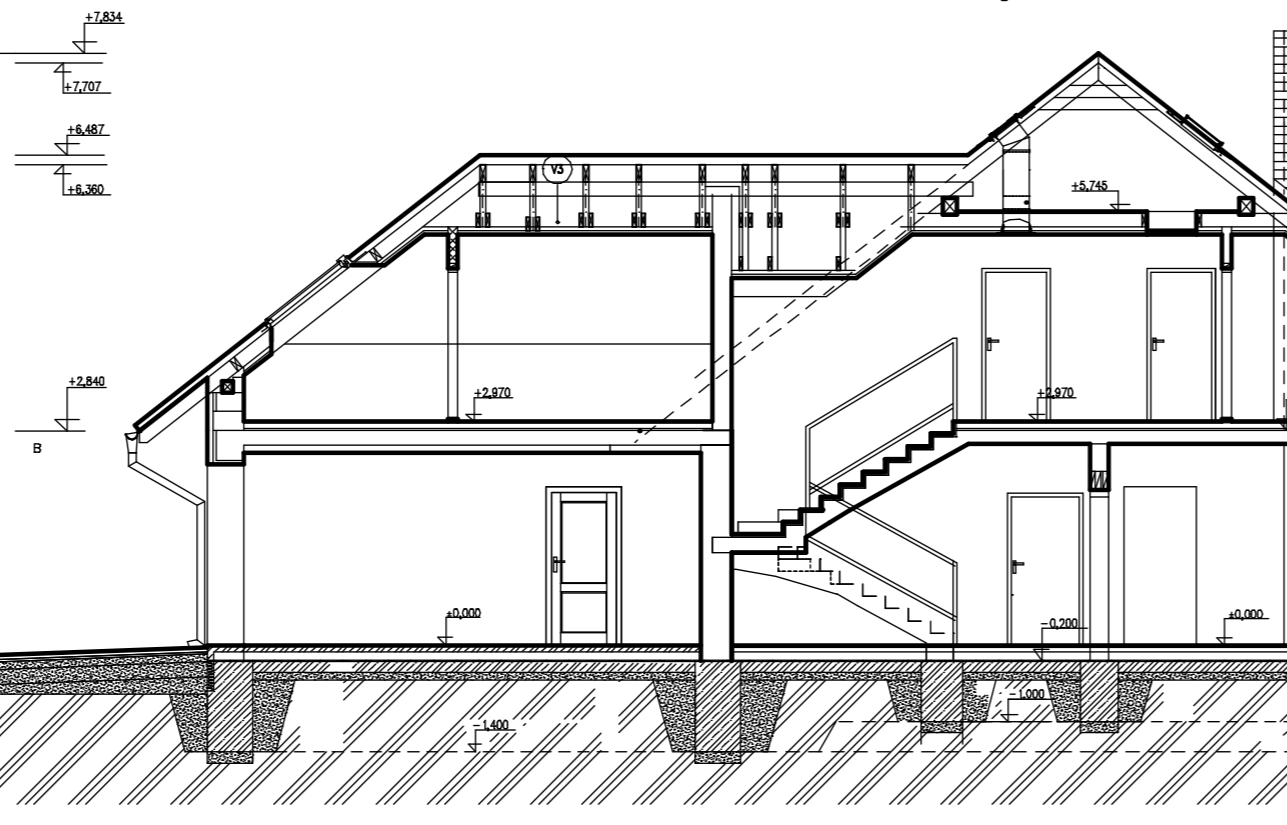
ŘEZ A-A:
