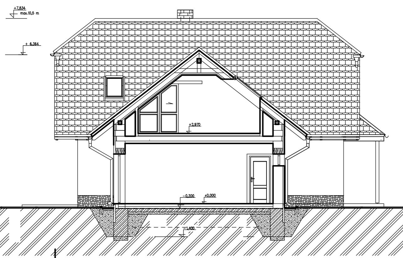
ŘEZ B-B:
