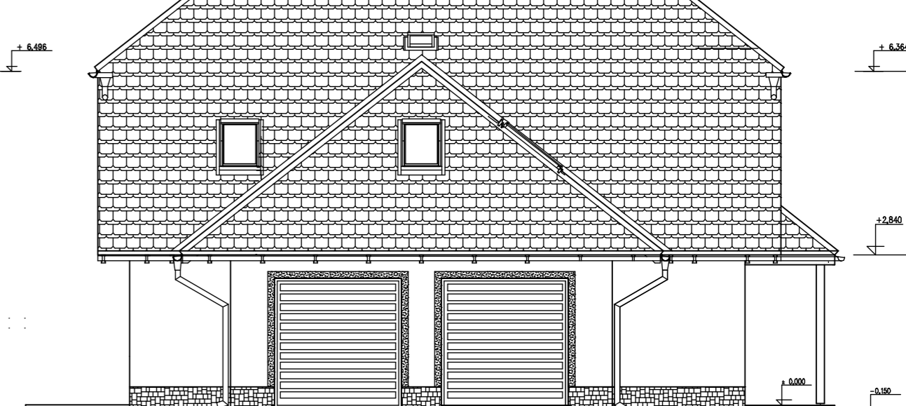
POHLED BOČNÍ 2:
